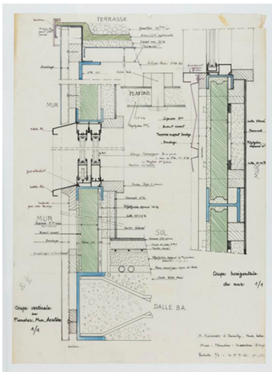
Plans en coupe des murs.
