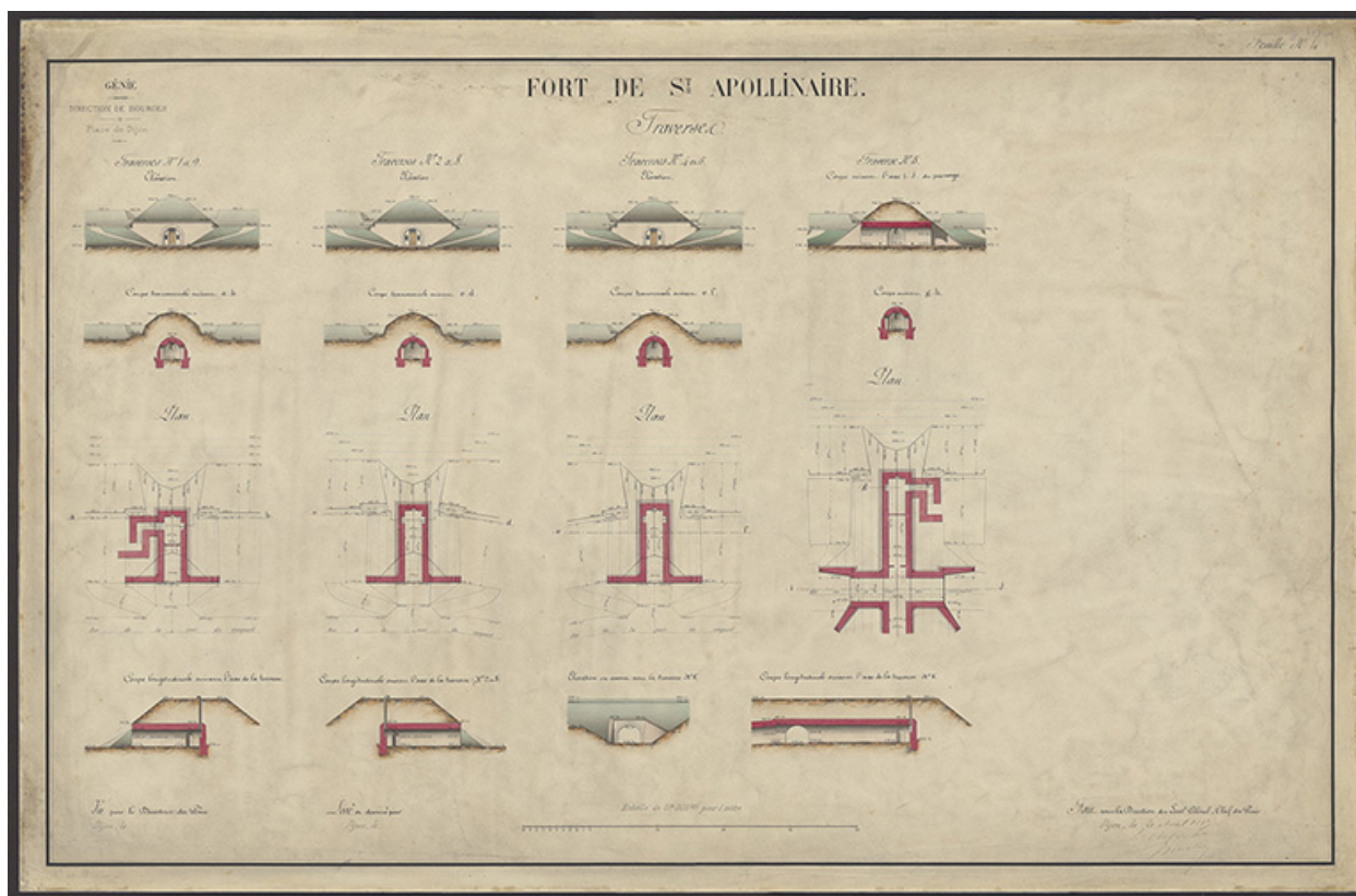
Fort de St Apollinaire. Traverses. 1885.
