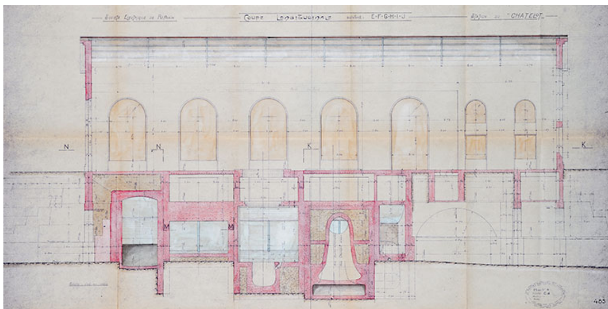
Société Electrique de Belchamp. Station du Chatelot. Coupe longitudinale de l'usine, pièce n° 11, 1934.
