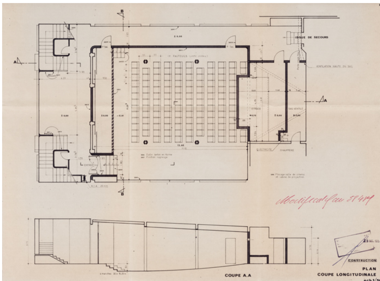
Société du Cinéma Alpha [aménagement d'une salle en sous-sol]. Plan, coupe longitudinale. 1975.
