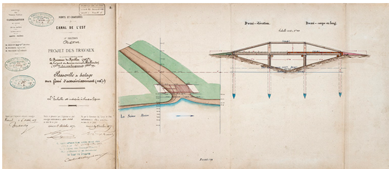
Passerelle de halage sur fossé d'agrandissement, 168k (1877).
