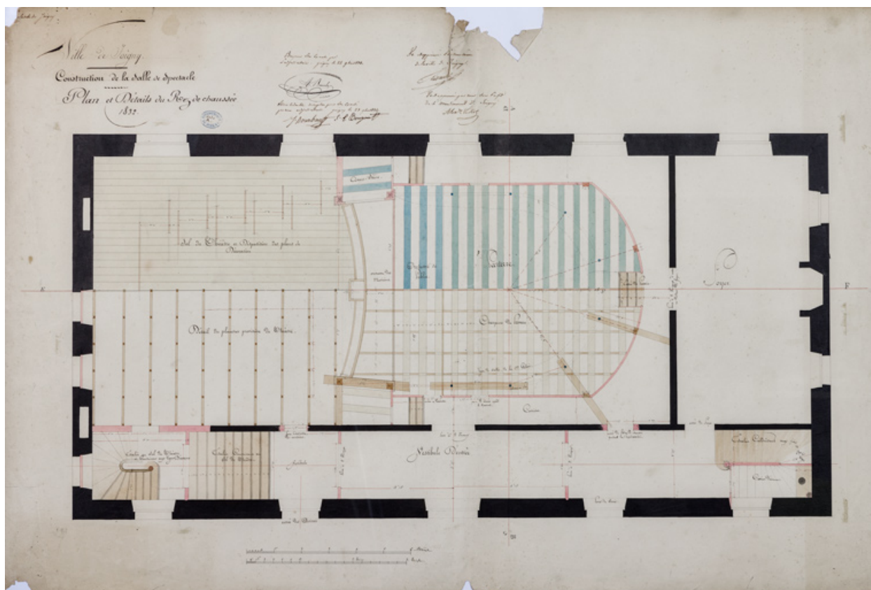
Construction de la salle de spectacle. Plan et détails du rez-de-chaussée. 1832.
