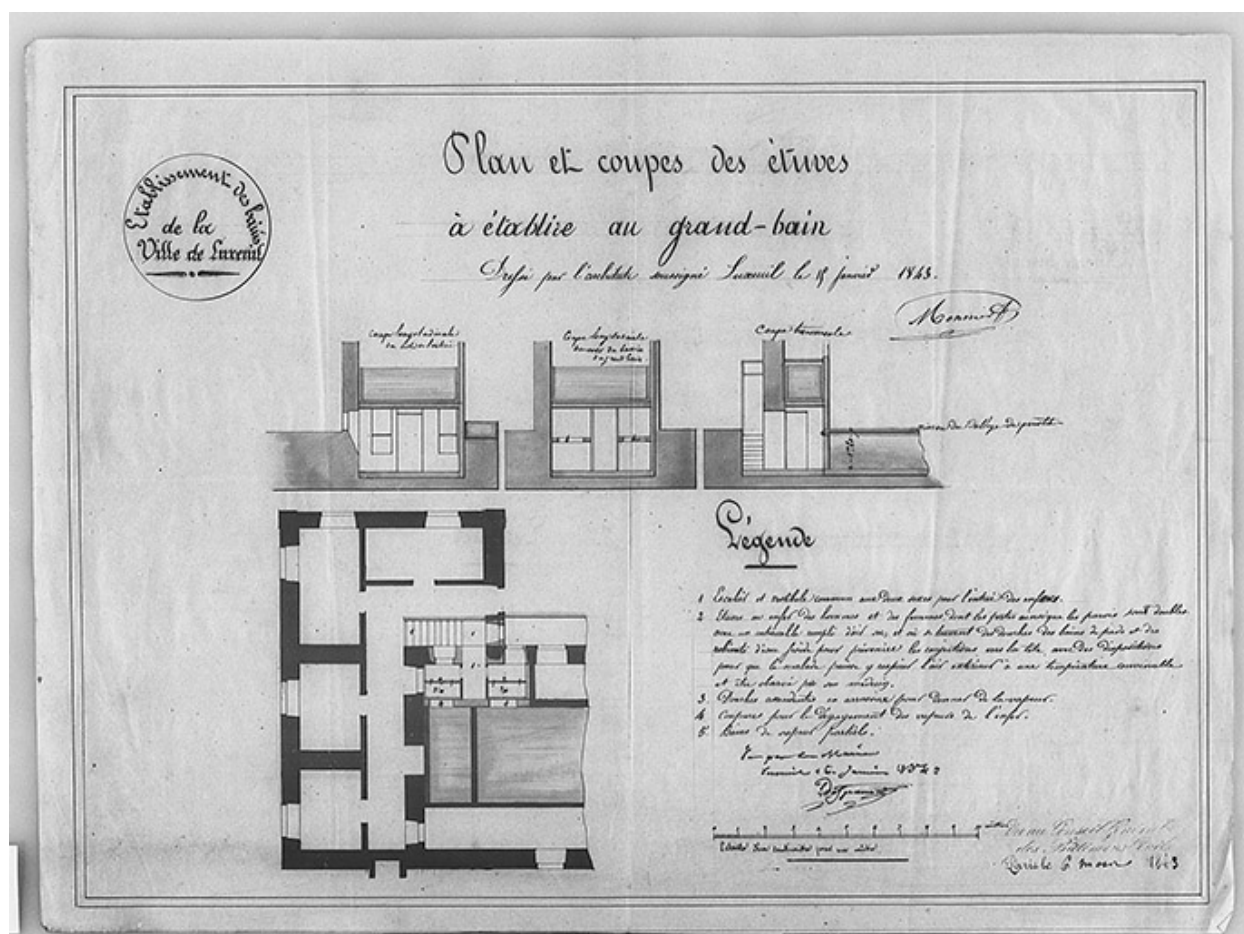
Projet de Bain spécial ferrugineux, plan et coupe sur les étuves (15 janvier 1843).
