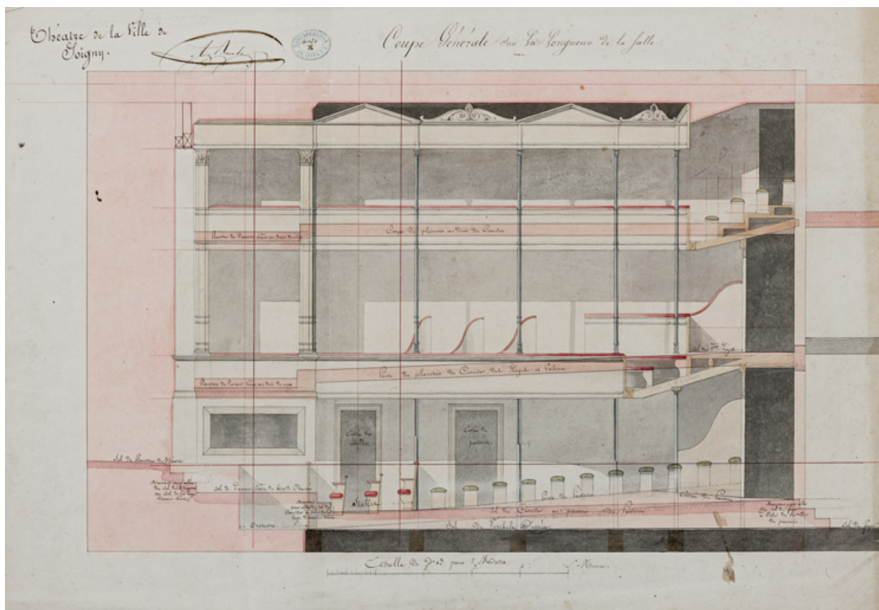
Construction de la salle de spectacle. Coupe générale sur la longueur de la salle. 1832.
