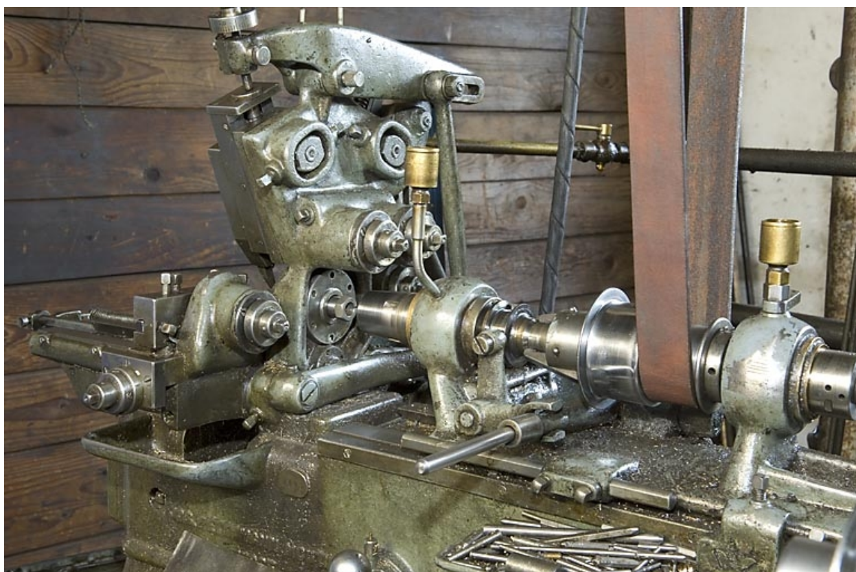
Tour à décolleter Petermann (M). Détail du système d'entraînement de la poupée mobile.
