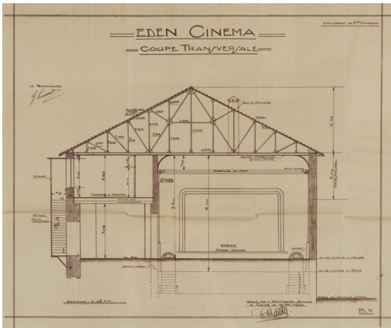
Eden-Cinéma. Coupe transversale. 1934.
