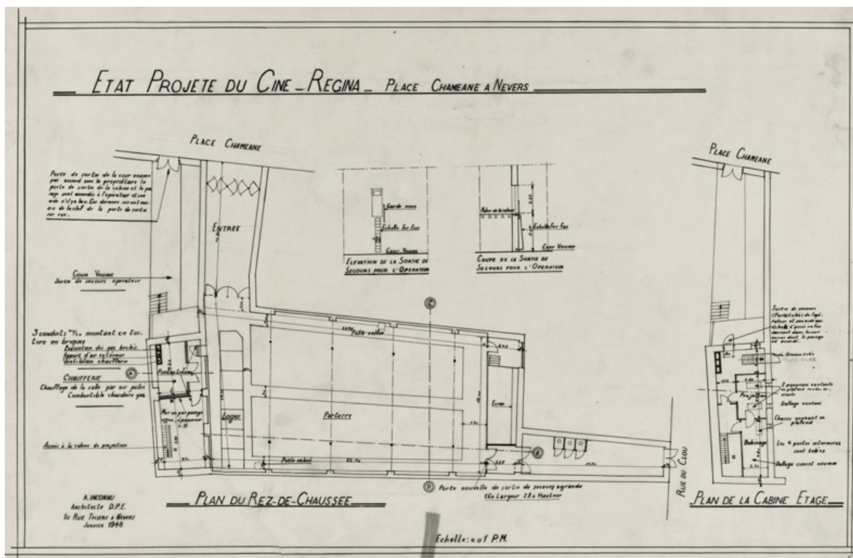
Etat projeté du Ciné-Regina. Place Chaméane à Nevers [plans]. Janvier 1948.
