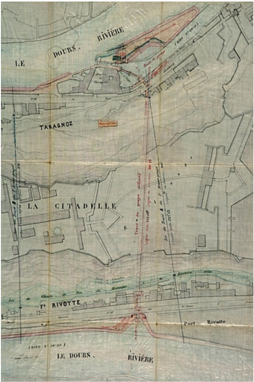
Dérivation sous la citadelle de Besançon. Plan de la dérivation et de ses abords [détail : tracé définitif, en rouge], 1877.
