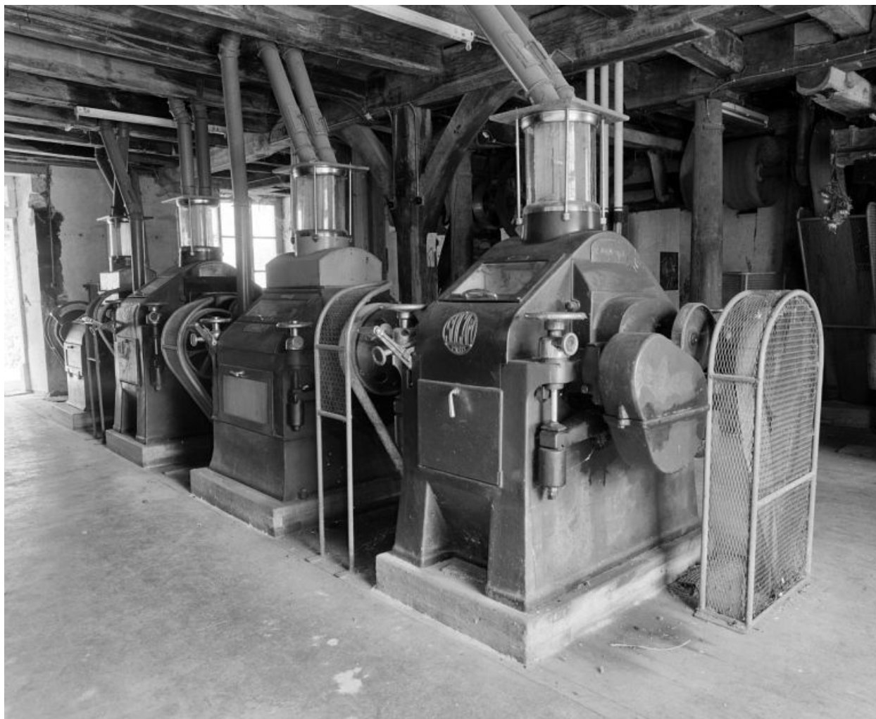
Rez-de-chaussée. Broyeurs.
