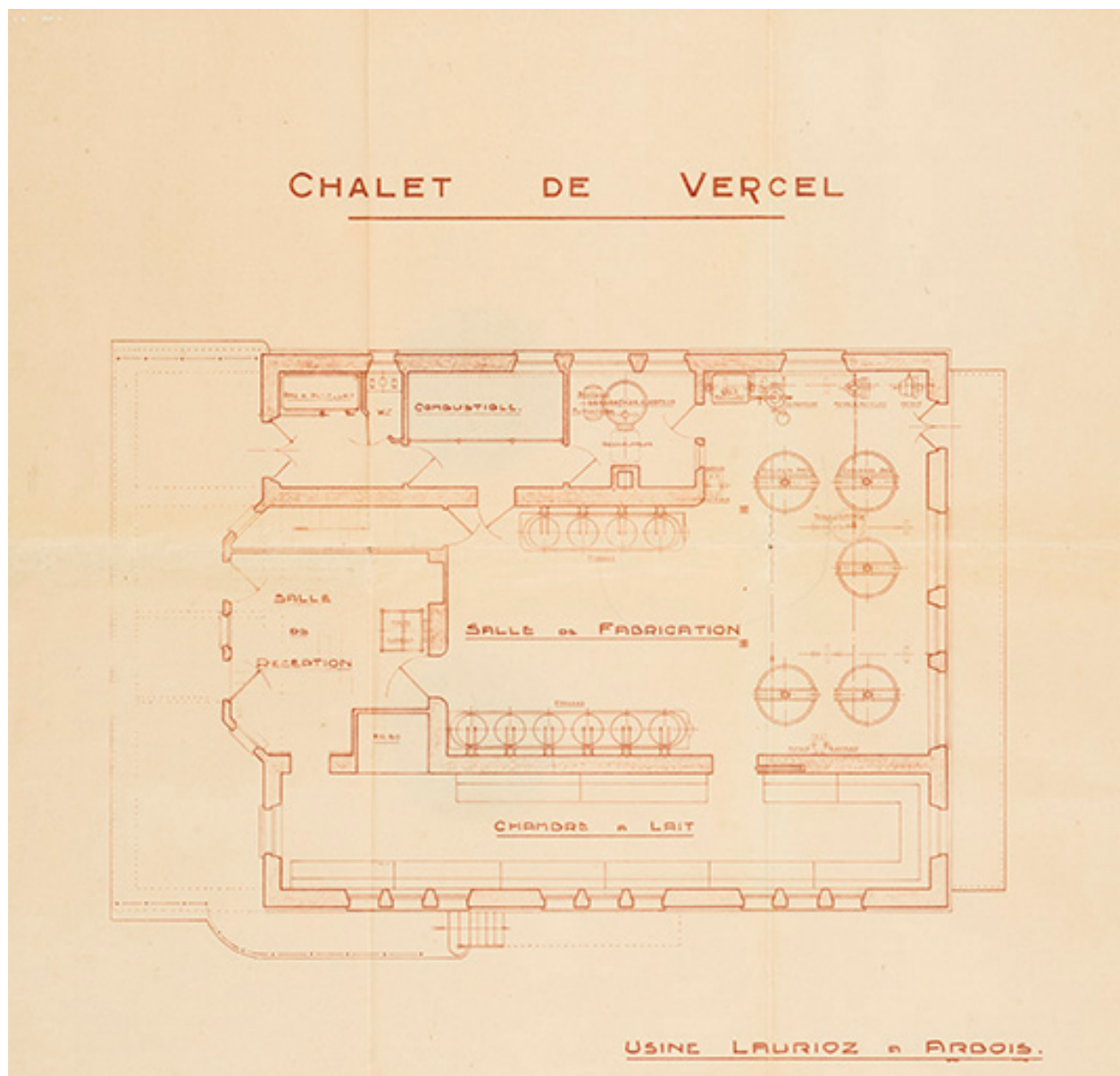
Chalet de Vercel. [Plan d'installation du matériel par la société Laurioz à Arbois], s.d. [1938]
