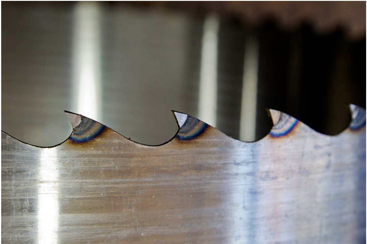
Atelier d'affûtage (K) : détail d'une lame de scie à ruban à double denture.
