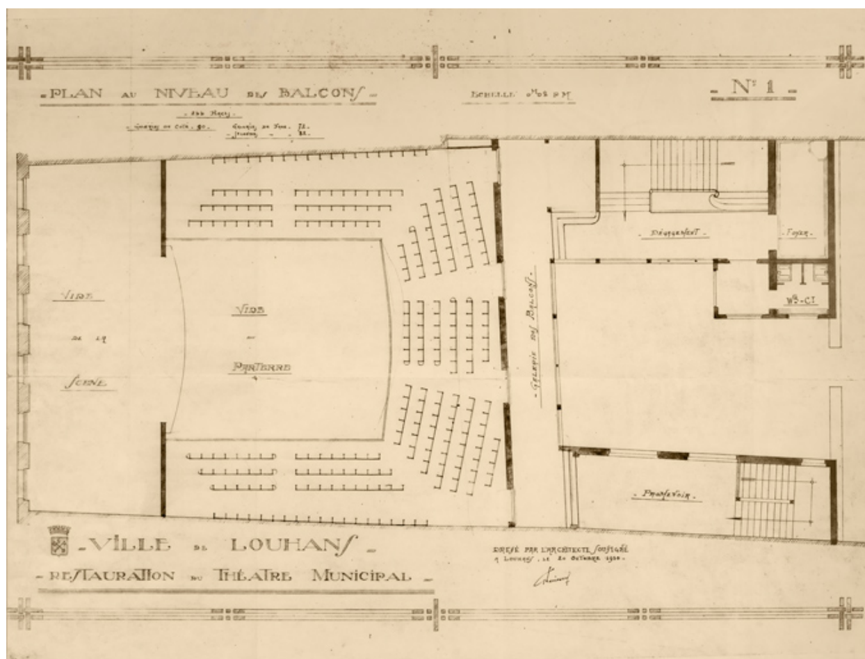
Ville de Louhans. Restauration du théâtre municipal. Plan au niveau des balcons. 20 octobre 1930.
