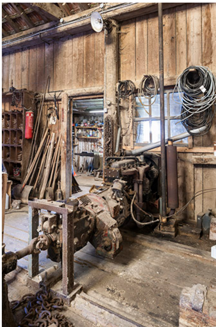
Moteur auxiliaire Saviem (au premier plan) et atelier d'affûtage.
