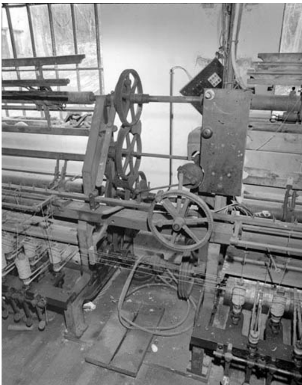
Système moteur.
