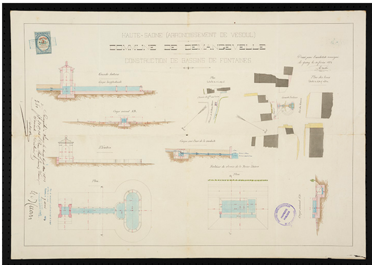
Plan : construction de bassin de fontaines. (1873)
