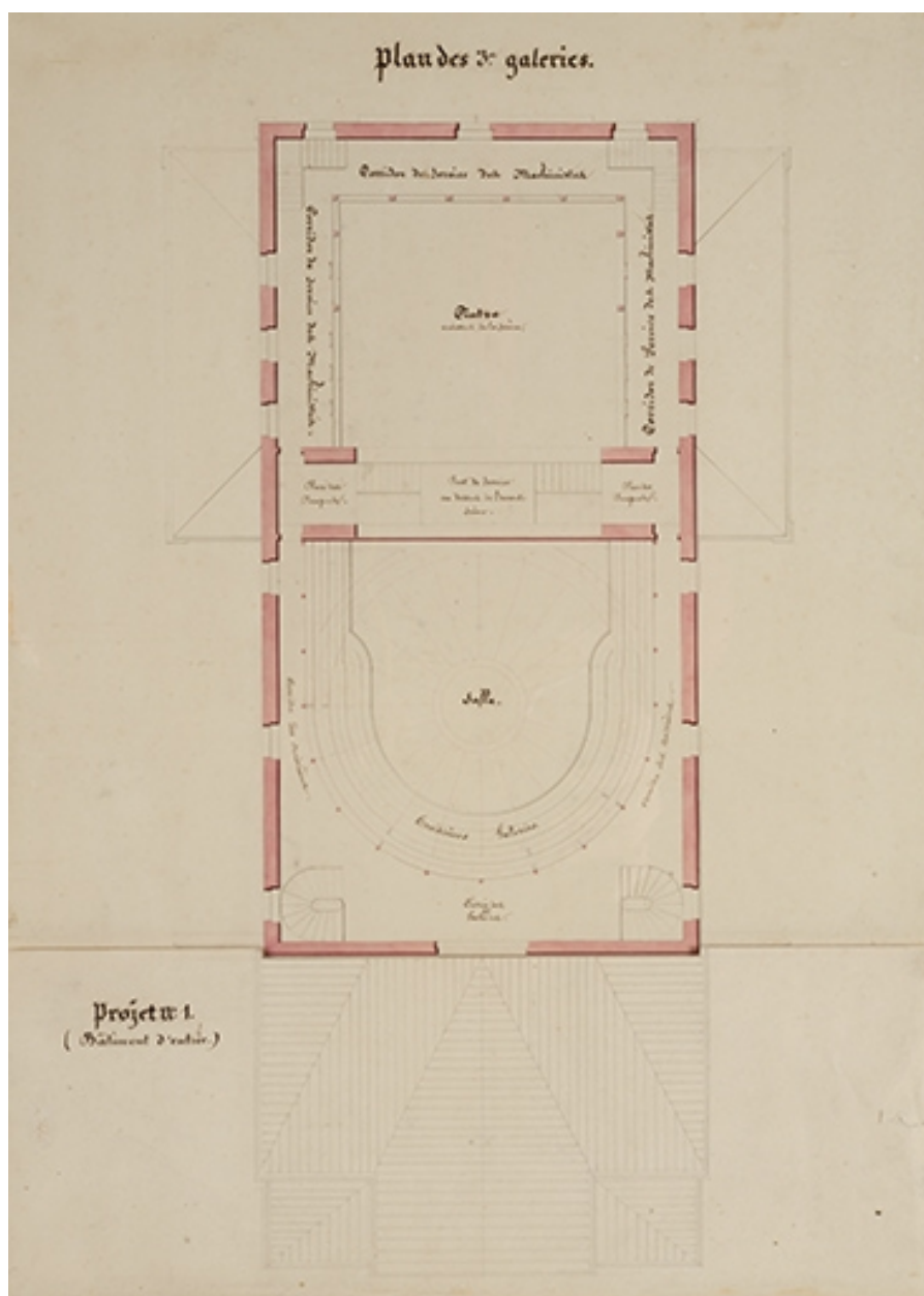
Théâtre de Dôle. Convenance, Economie [projet H]. Plan des 3e galeries. En bas : Projet n° 1 (Bâtiment d'entrée). S.d. [1839].
