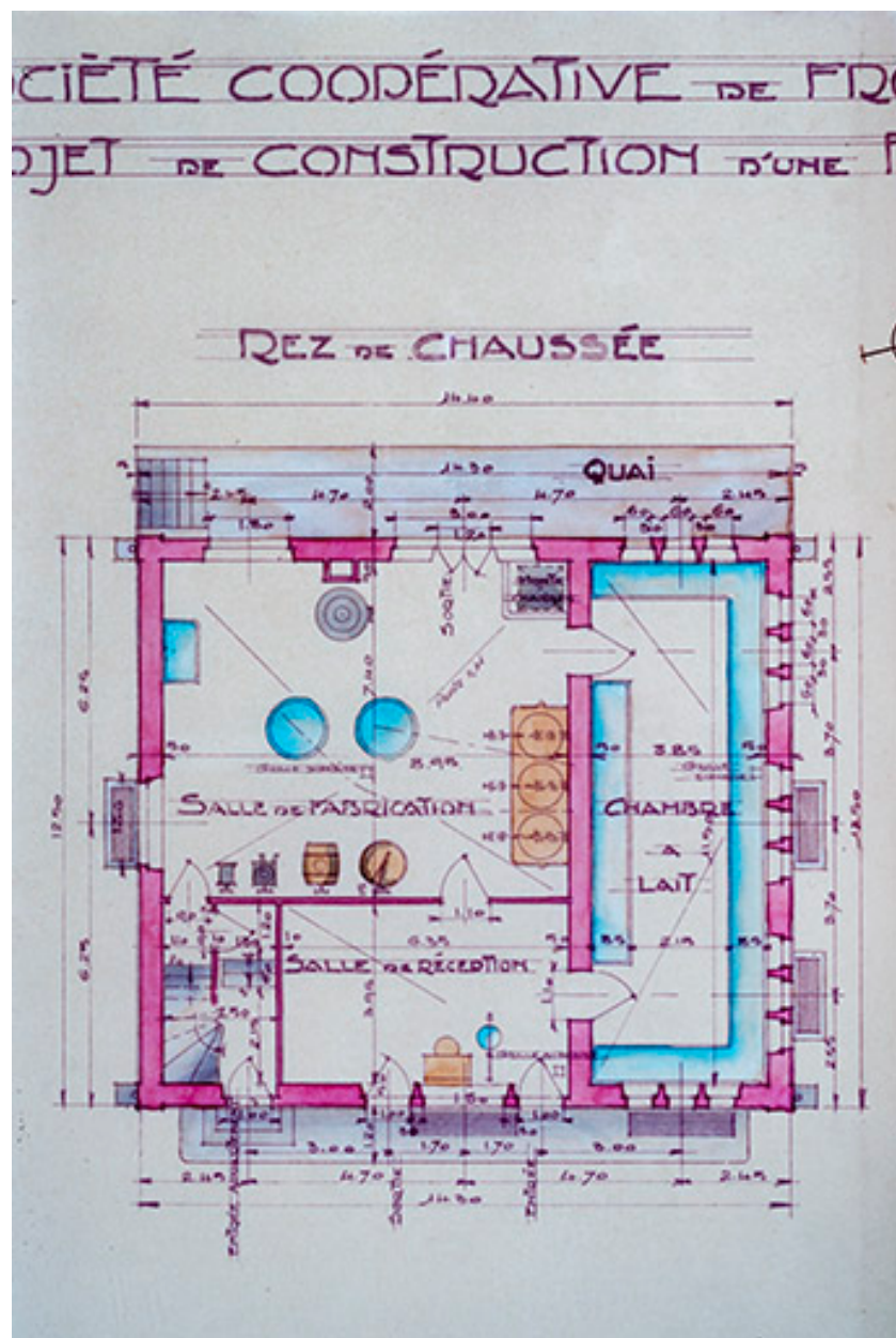
Société coopérative de fromagerie. Avant-projet de construction d'une fromagerie - Plan du rez-de-chaussée, 1929.
