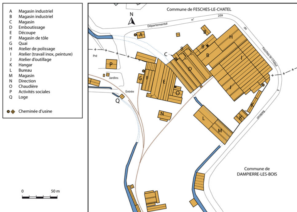
Plan-masse de l'usine en 1977. D'après un extrait du plan cadastral.
