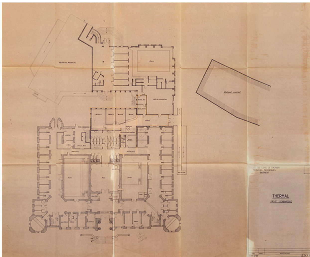
Plan du rez-de-chaussée, projet (24 septembre 1990).
