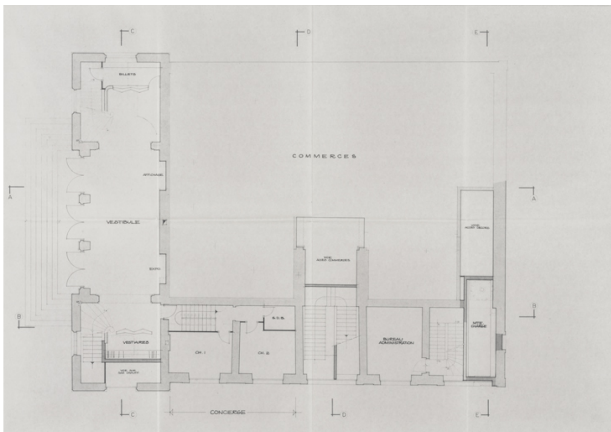
Ville d'Autun. Théâtre municipal. Place du Champ de Mars. Projet de rénovation. 7706 14. Niveau vestibule. S.d. [1978 ?].
