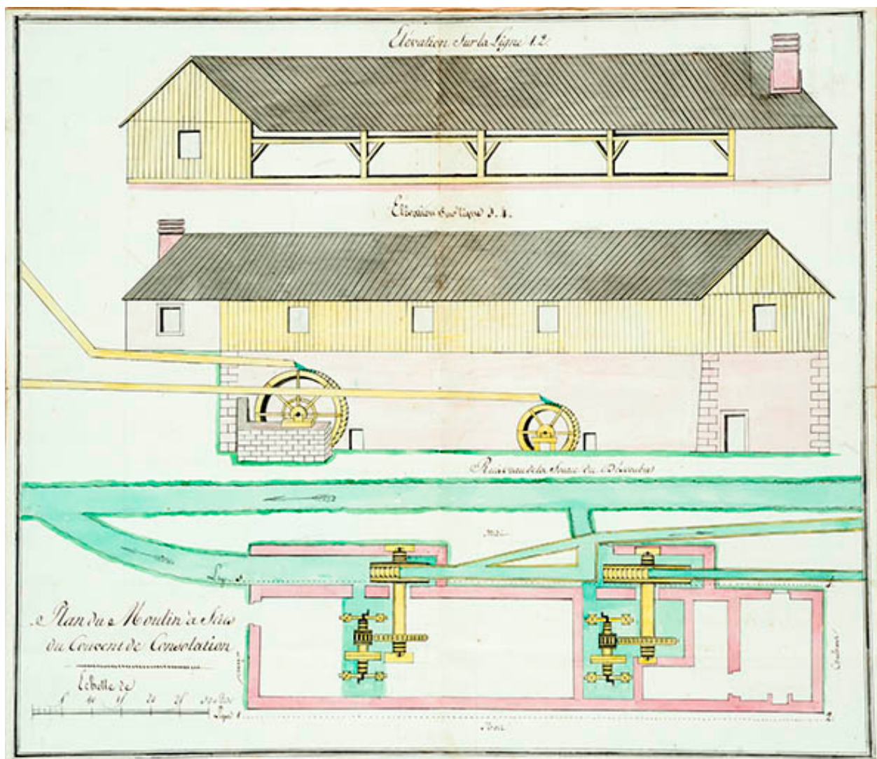
Scierie, Consolation-Maisonnettes (Val de Consolation) : plan du moulin à scies du couvent de Consolation, s.d. [vers 1820].
