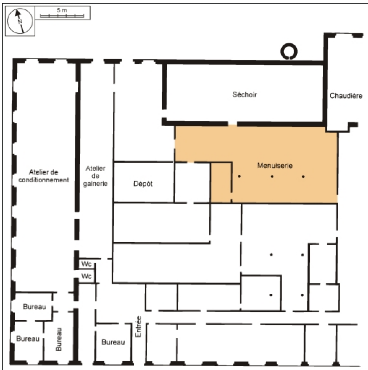
Plan de situation de l'atelier de menuiserie.
