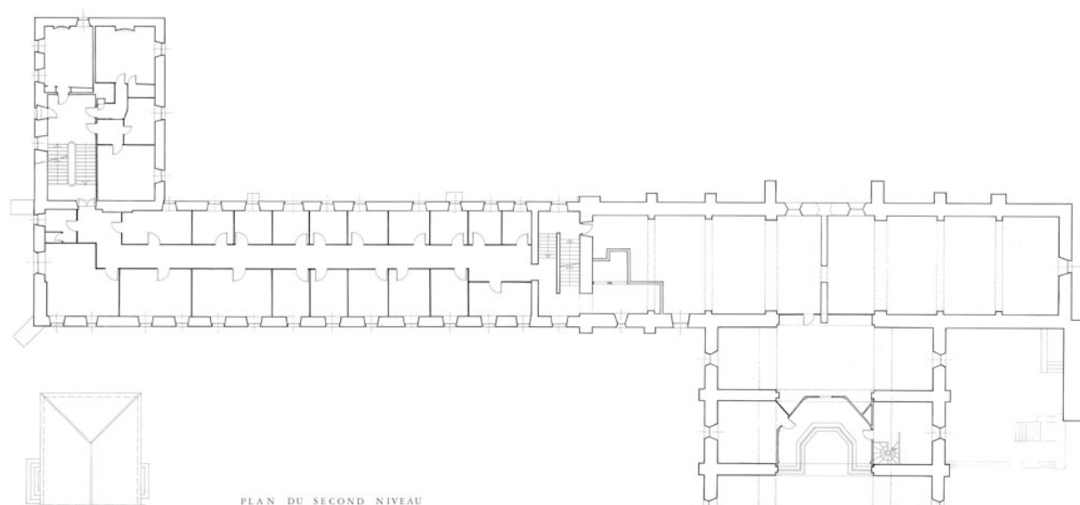
plan du second niveau
