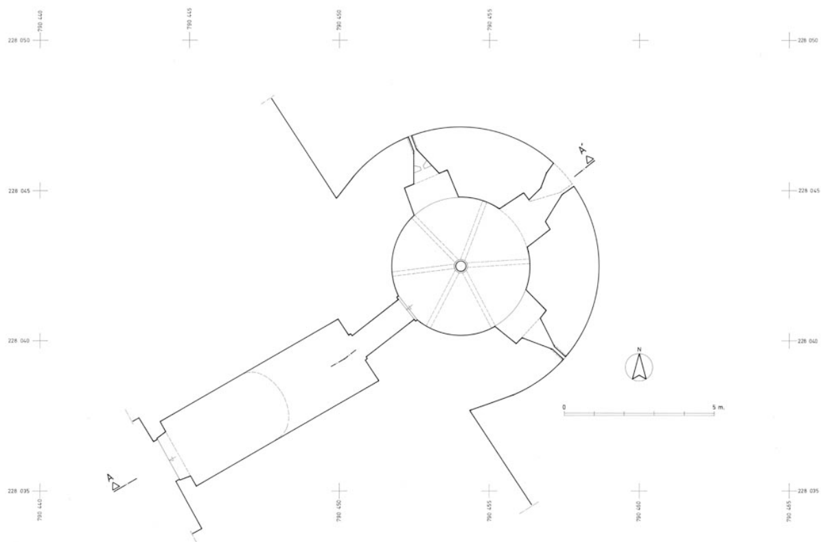
Tour Blondeau : plan du niveau inférieur.
