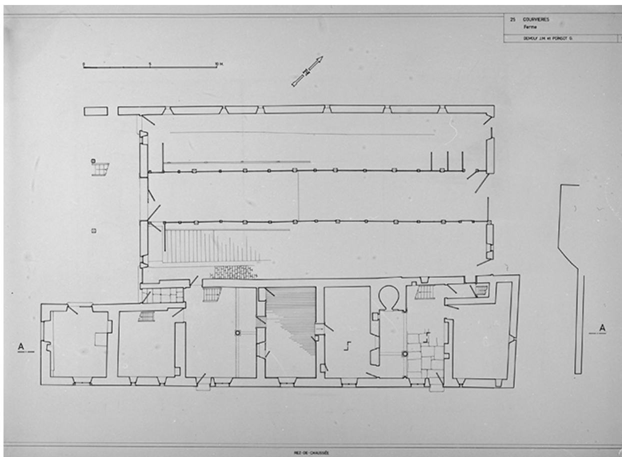
Plan au sol d'une ferme..
