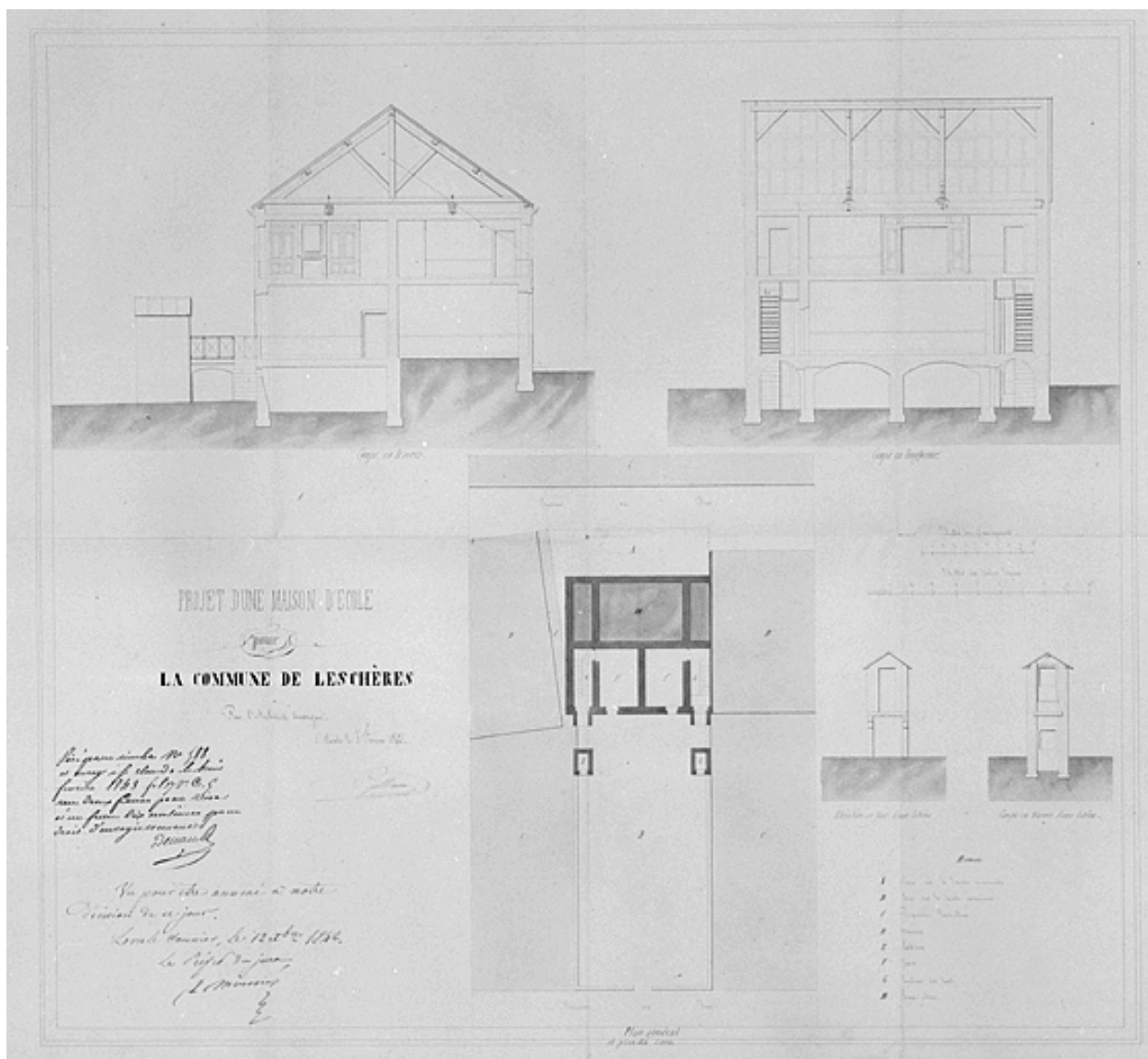
Projet d'une maison d'école pour la commune de Leschères [plan-masse et coupes].
