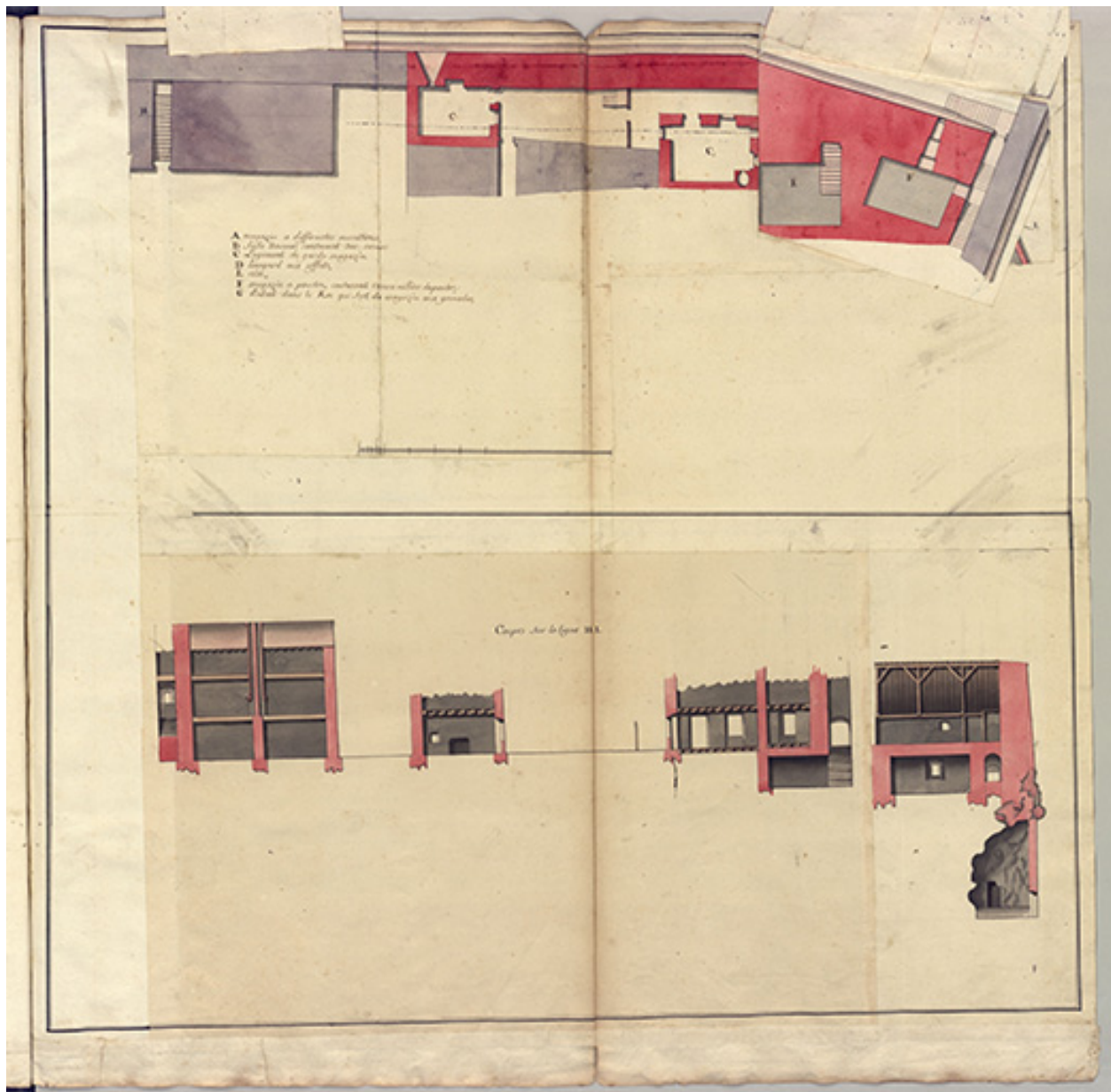
Fol. 16 Fort-Belin-sur-Salins : plans et coupes (magasin pour 12,000 milliers de poudre) - vue 2.
