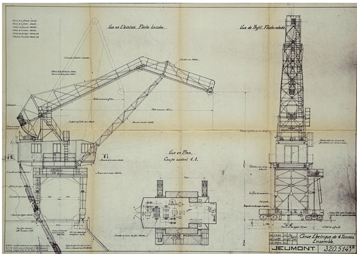
Grue électrique de 4 tonnes. Ensemble, 1936.
