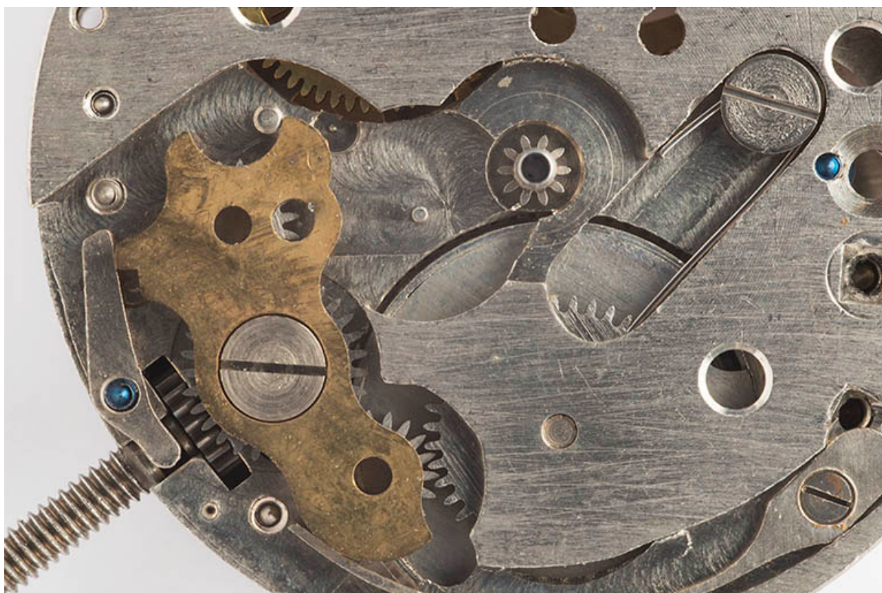
1er mouvement, côté cadran : détail du mécanisme du remontoir. A gauche, tige de remontoir et son pignon, et plaque protégeant les renvois.
