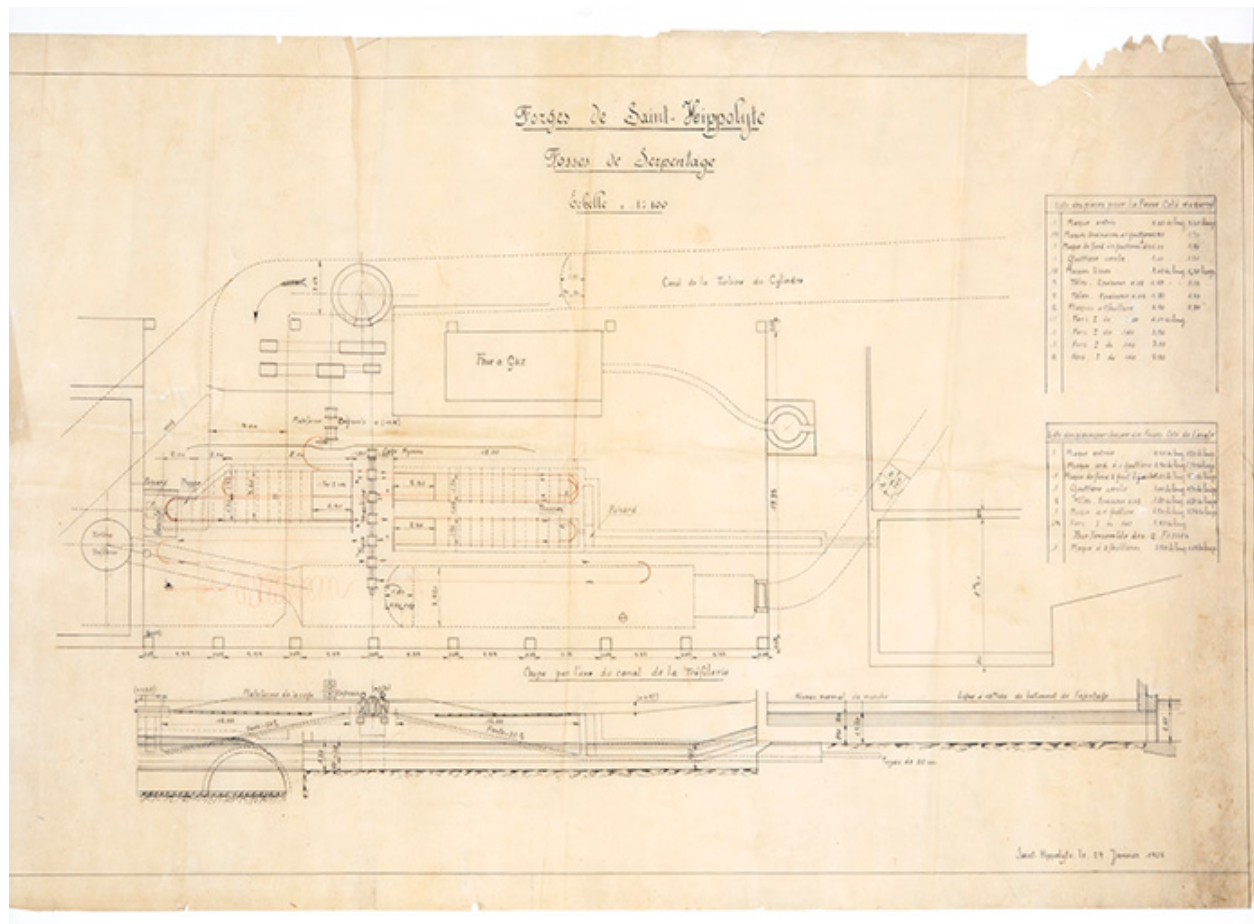
Forges de Saint-Hippolyte. Fosses de serpentage, 29 janvier 1925.
