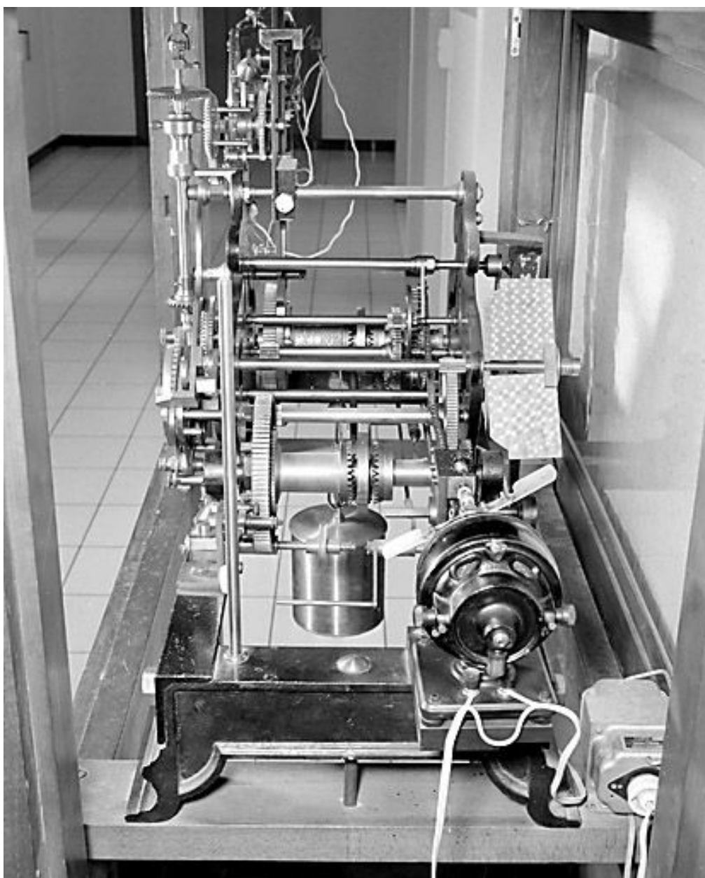
Vue d'ensemble du mouvement, de côté.
