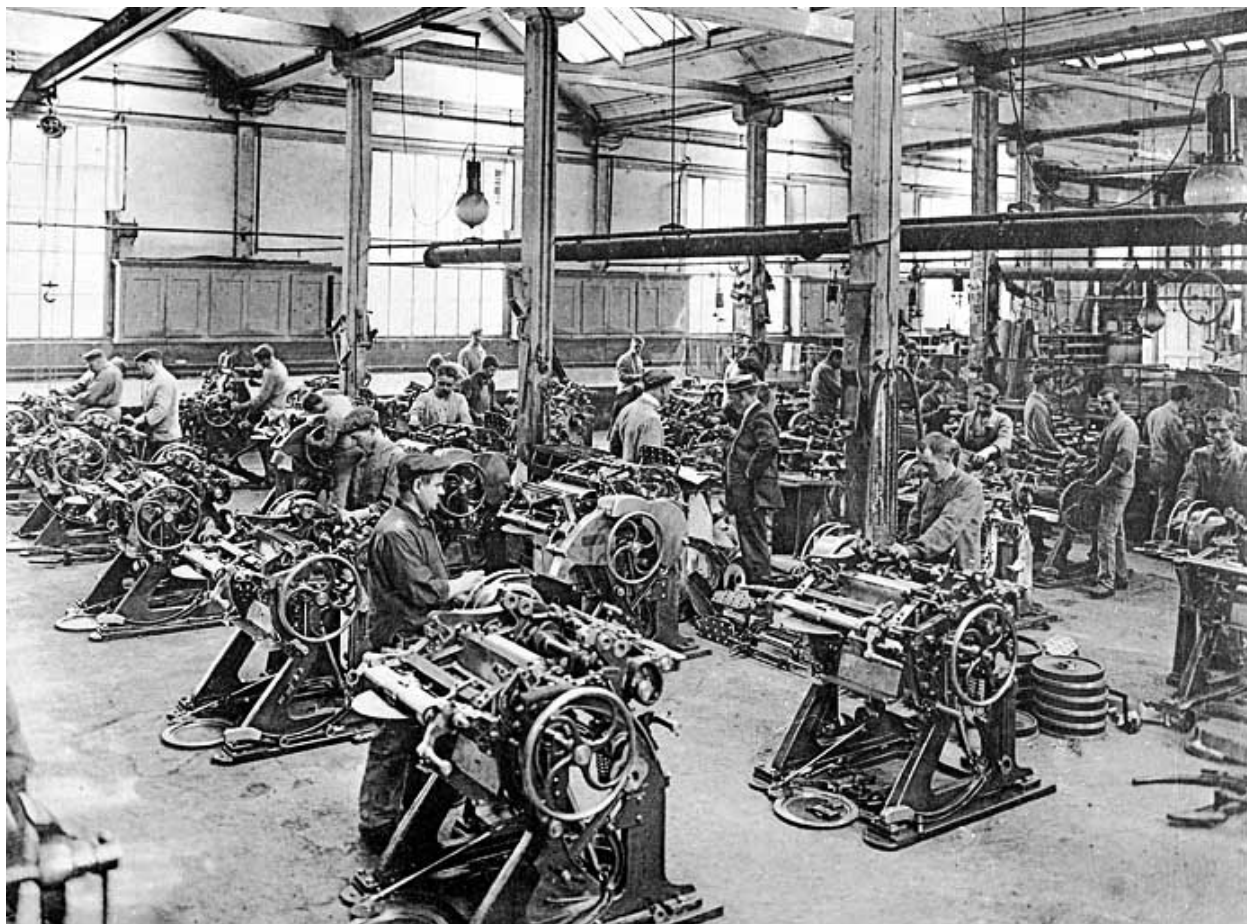
Montage des peigneuses.
