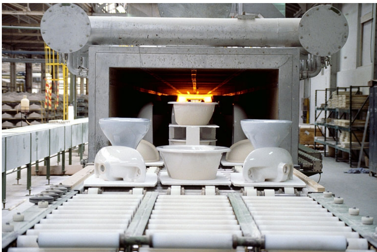
Usine de porcelaine Idéal Standard, Dole : défournement en bout du four tunnel.
