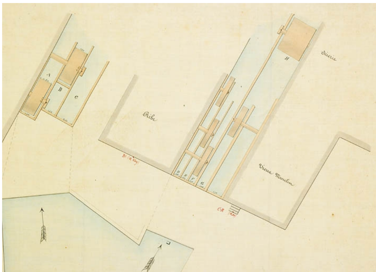
Plan de la tête d'eau et élévation des ouvrages [Plan-masse].
