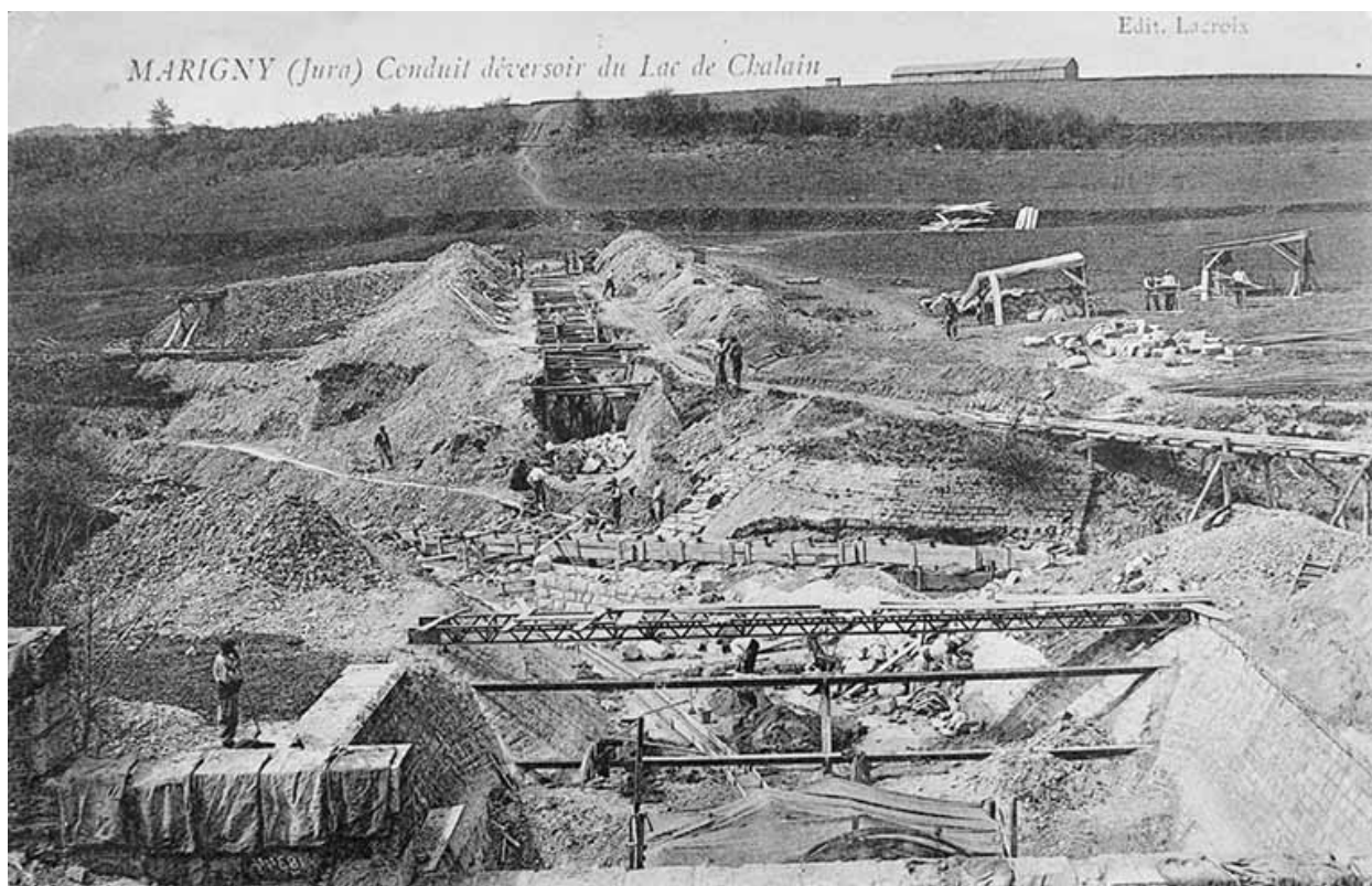
Marigny (Jura). Conduit déversoir du Lac de Chalais [le chantier vu depuis le haut de la conduite].
