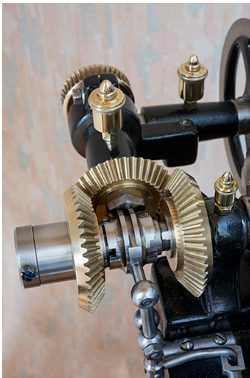
Engrenages et transmission du module de commande.
