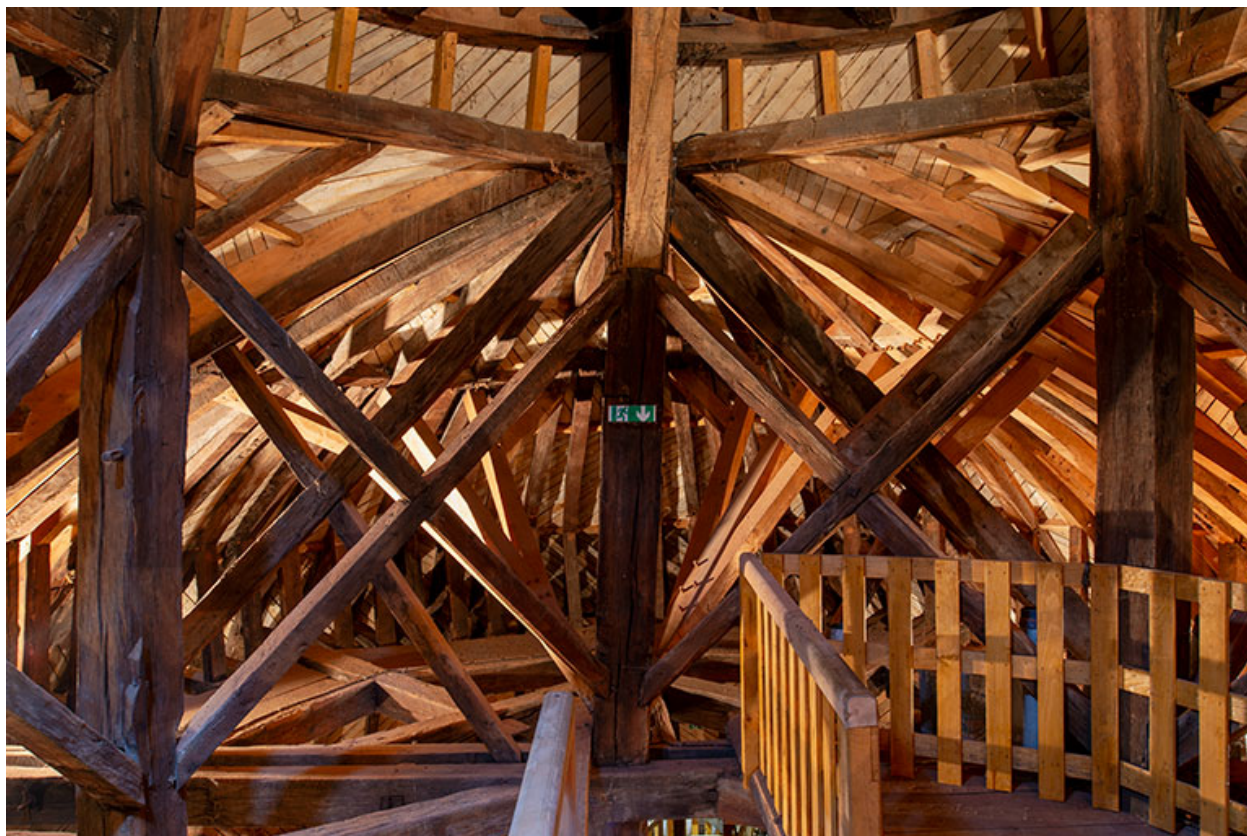
Partie orientale de la charpente, depuis le niveau intermédiaire. Vue axiale.
