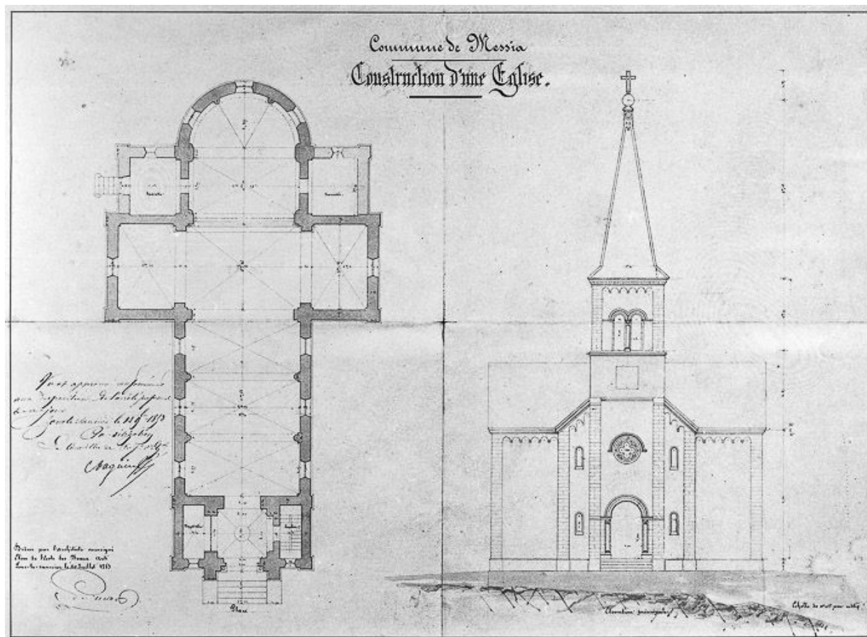
Plan, élévation principale.
