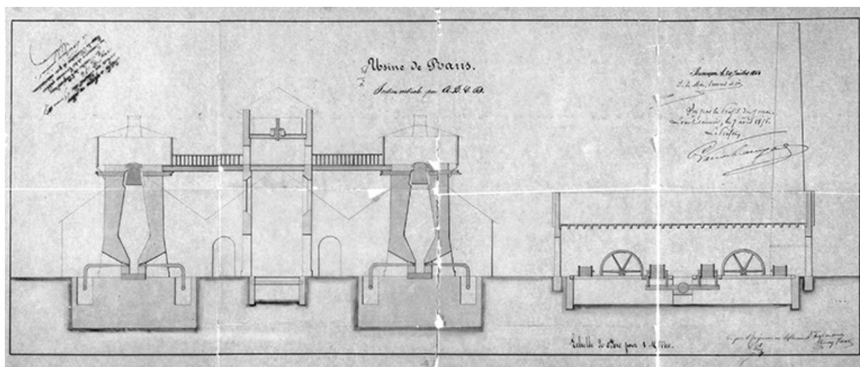
Usine de Rans. Section verticale par A.B.C.D.
