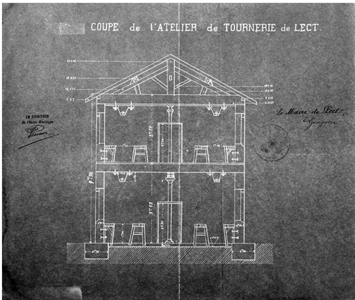
Atelier de tournerie à Lect. Coupe.
