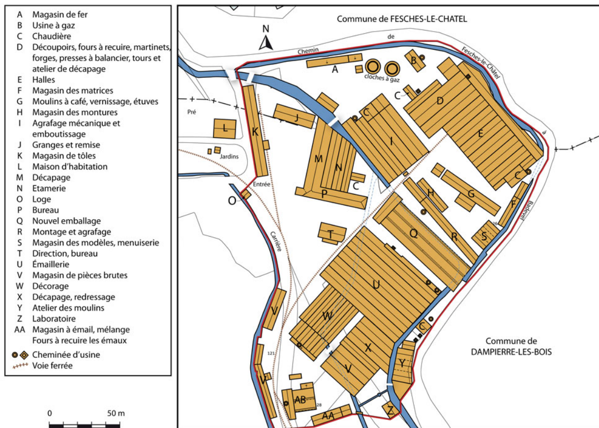
Plan-masse de l'usine en 1895. D'après le plan général de la Casserie, 1895.
