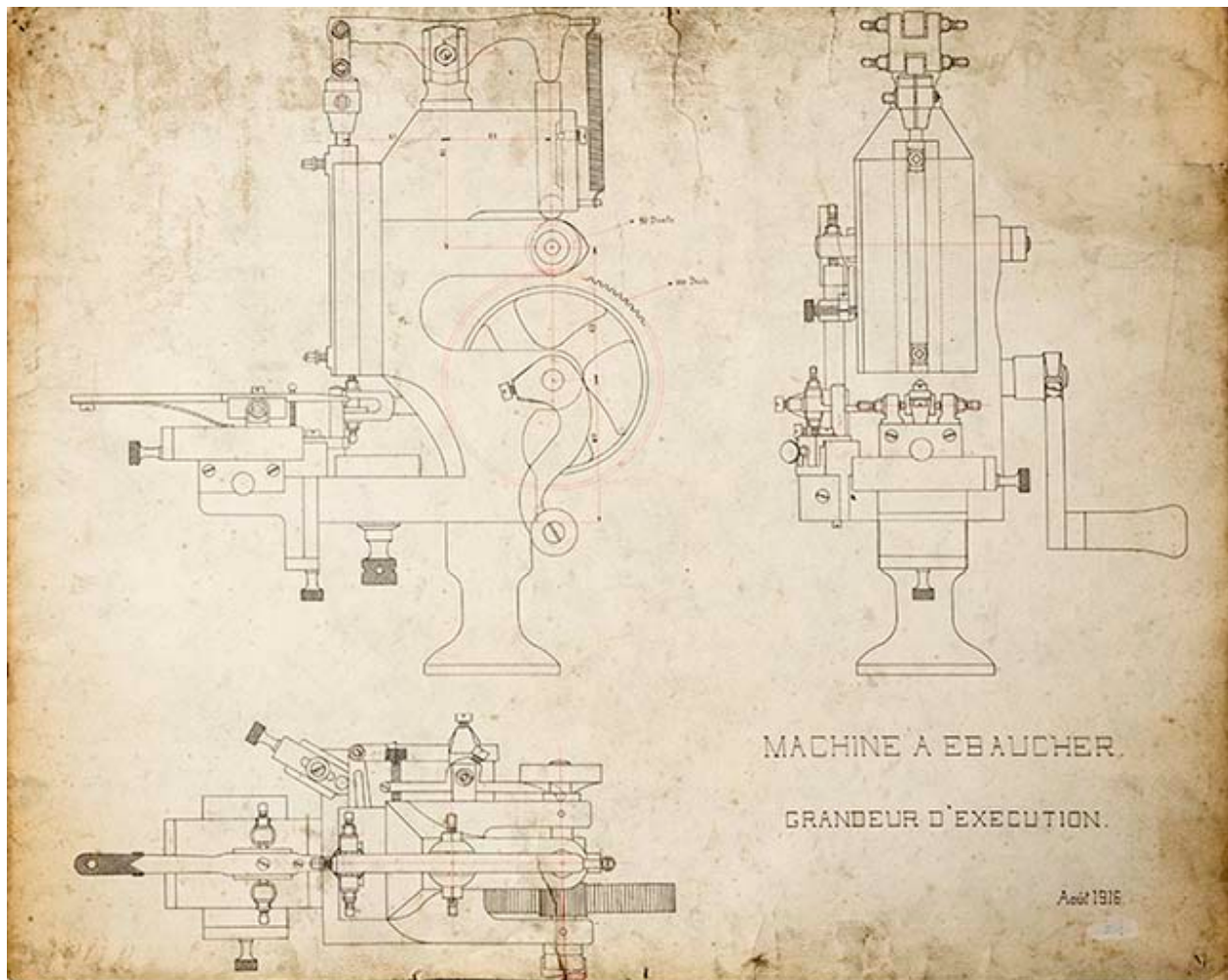
Machine à ébaucher. Grandeur d'exécution, août 1916.
