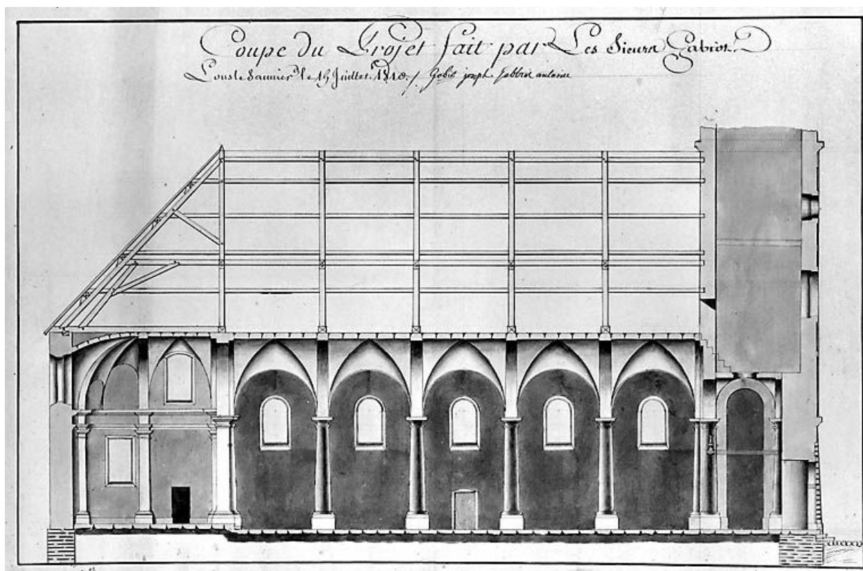
Coupe du projet fait par les sieurs Gabiot, 1810. Dessin (plume, lavis), 15 juillet 1810, sans échelle.
