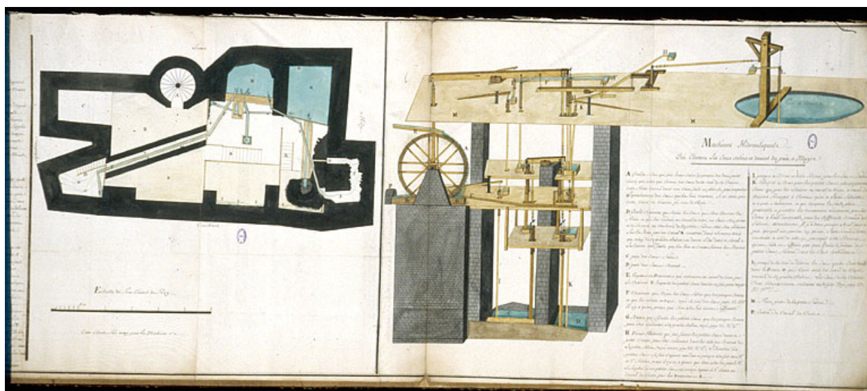
Machines Hydrauliques Qui Elèvent Les Eaux salées et douces du puits à Muire, 1756.
