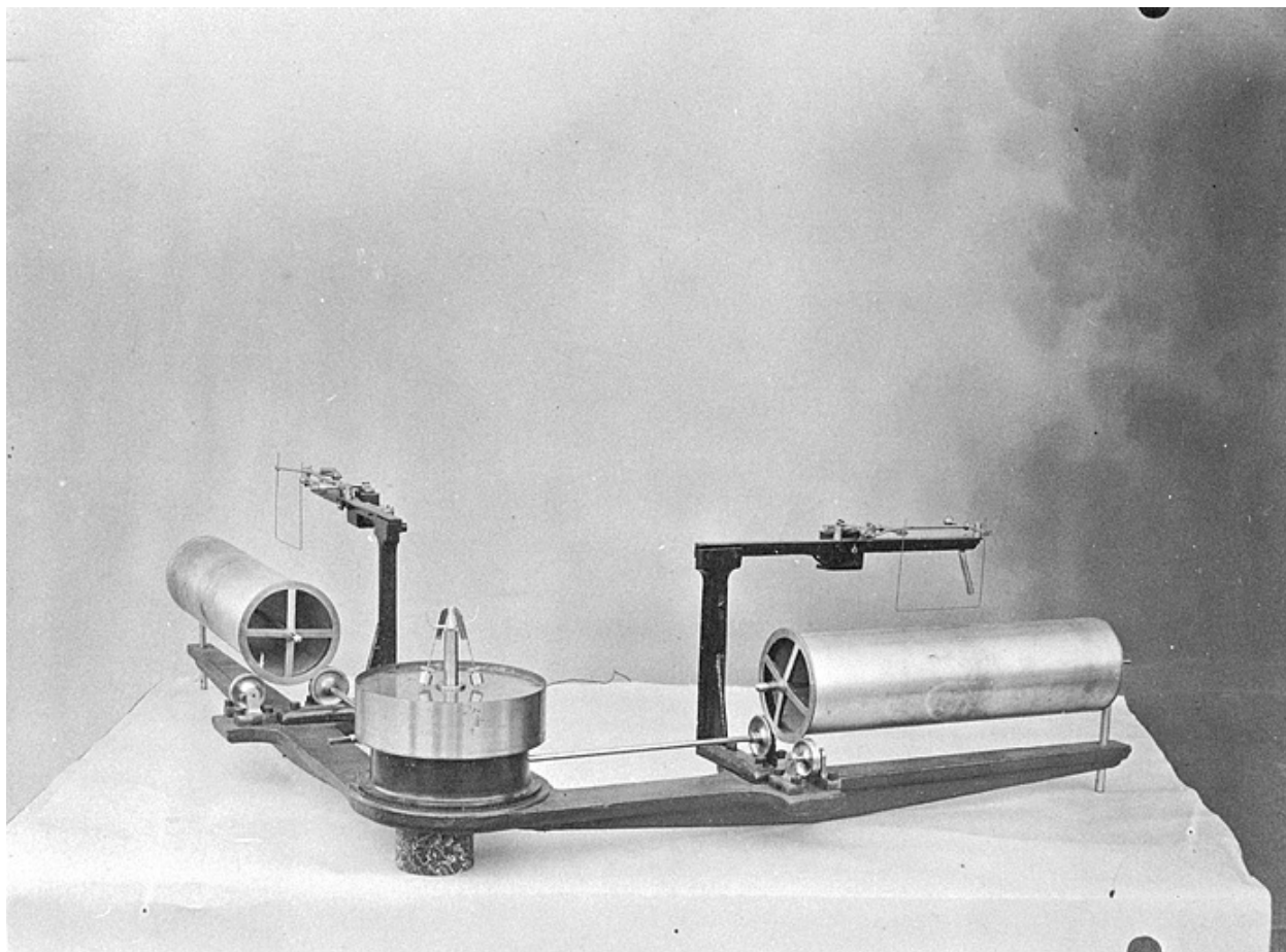
[Enregistreur du sismographe Mainka-Bosch], 1911.
