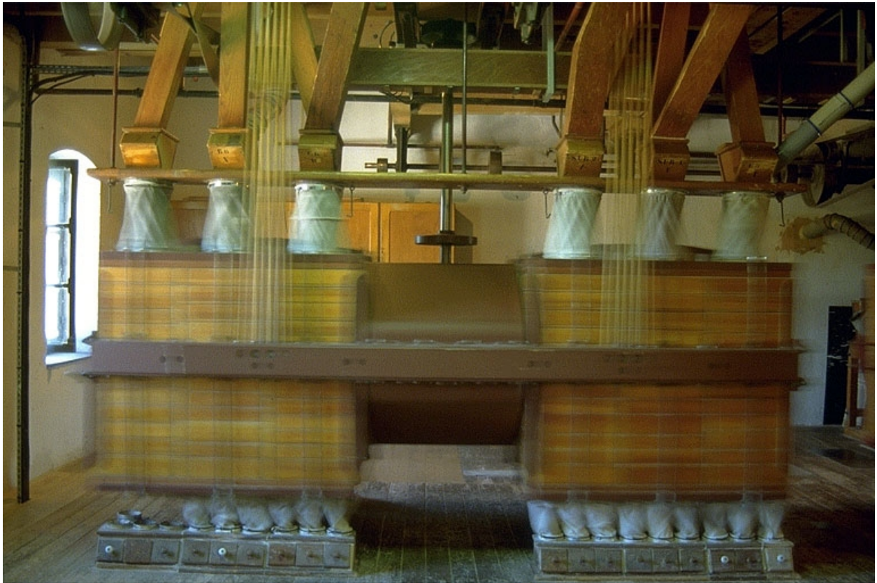
Atelier de fabrication (L), 3e étage : plansichter en fonctionnement.
